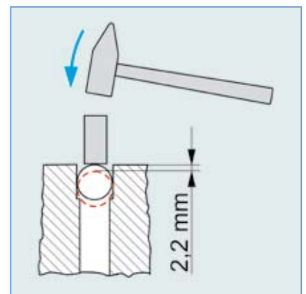
Abb. 2 Montage der Kugel am Zylinderkopf [© MS Motor Service International GmbH]
